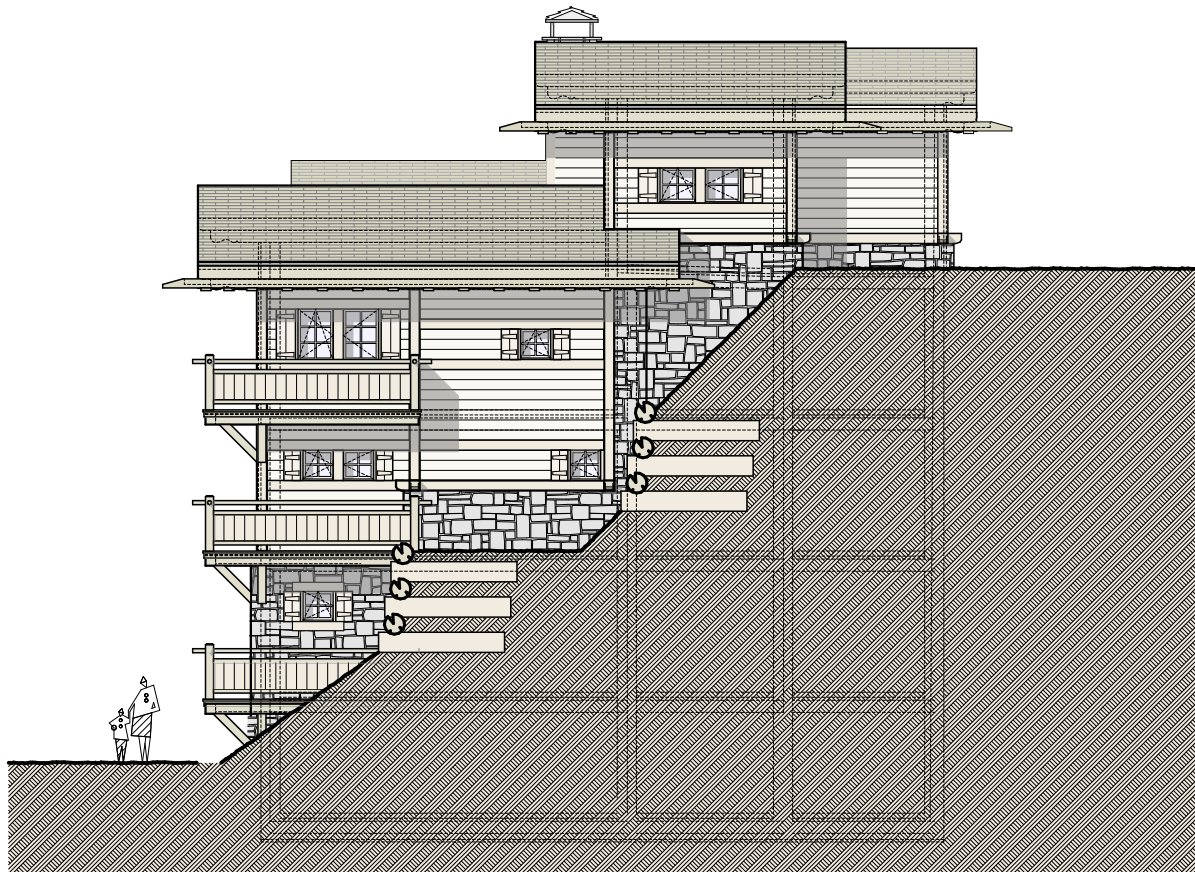
Façade Ouest
