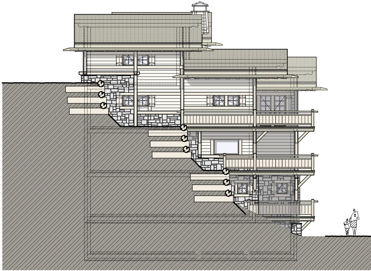
Façade Sud
