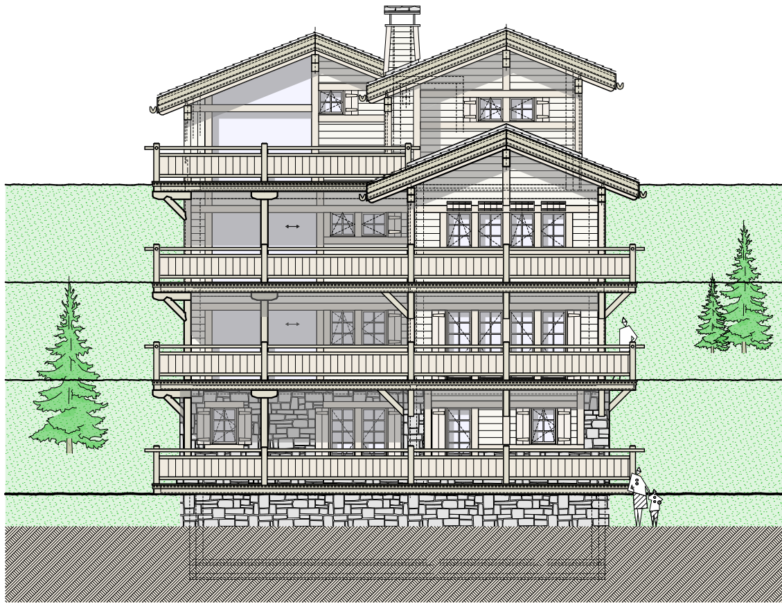
Façade Est
